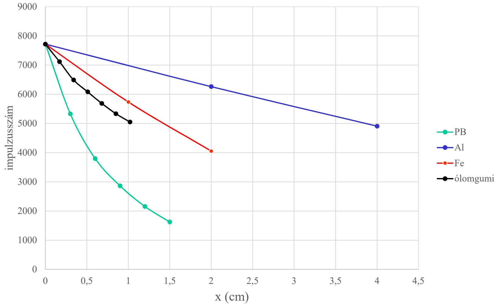
A ^{137}\text{Cs} gamma sugárzásának elnyelődése különböző anyagokban
