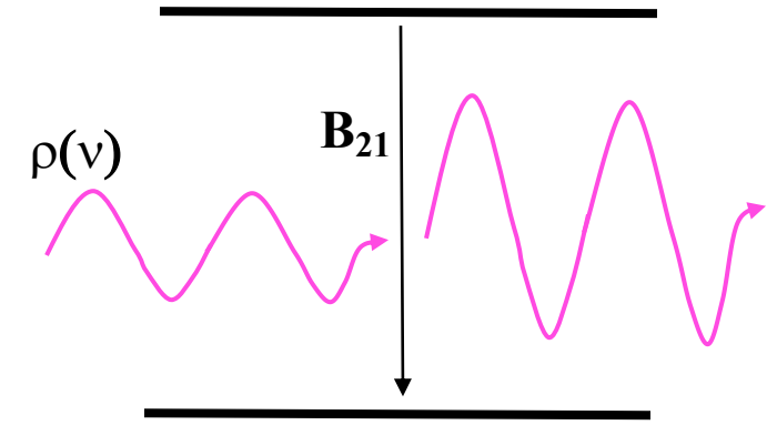
3. Indukált emisszió
