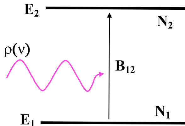
1. Abszorpció
