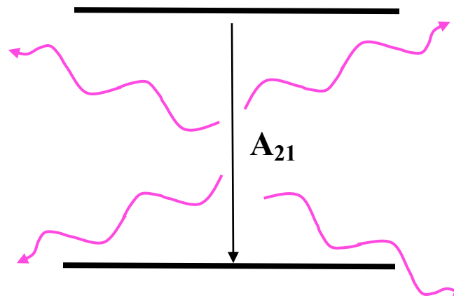
2. Spontán emisszió
